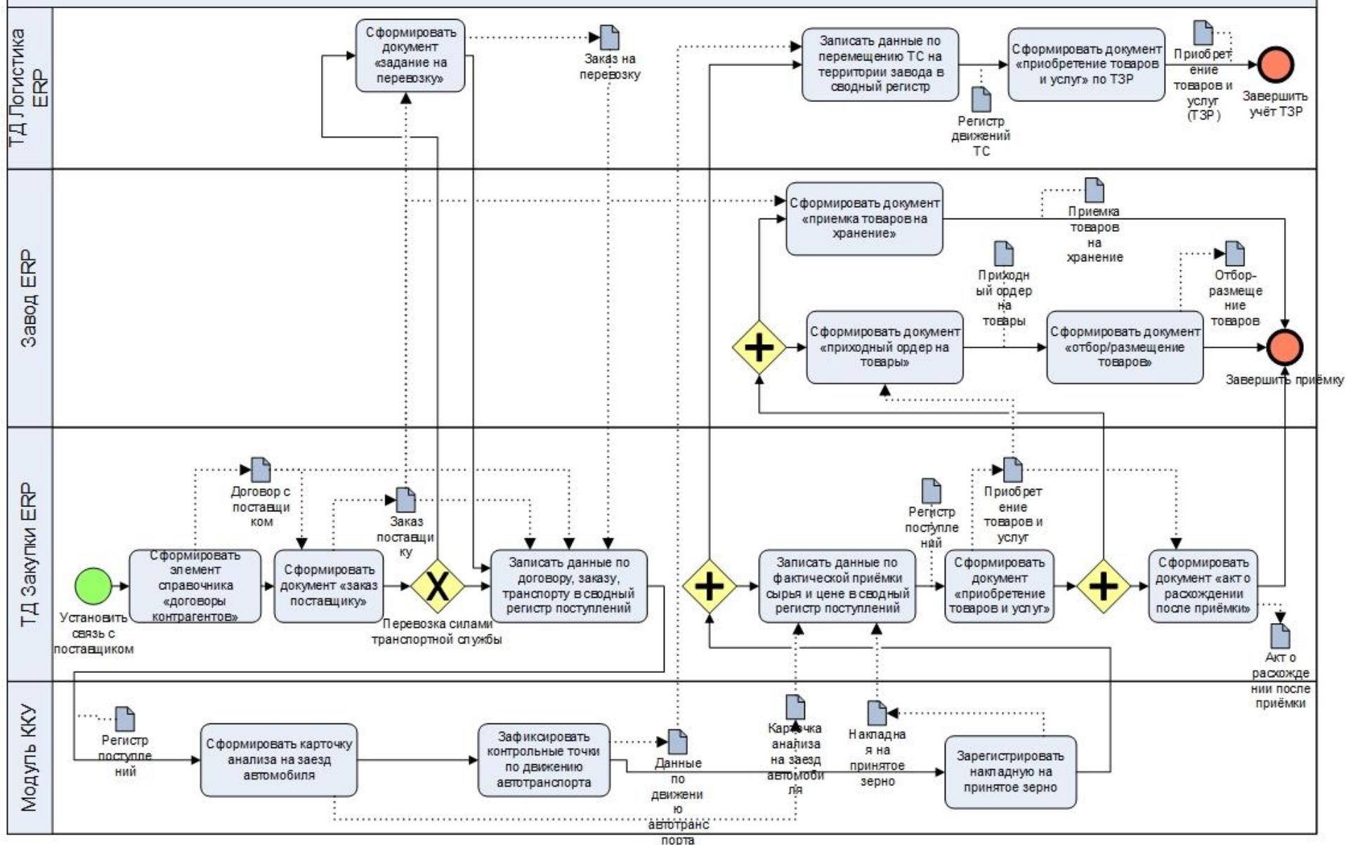
Приложение 4. Схема обмена с ПК «Зерно» (Закупка-приемка)
