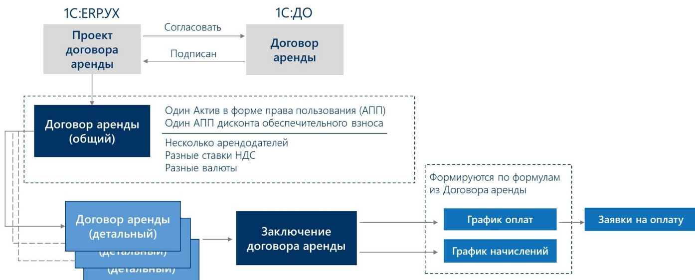
Схема 4. Измененная схема учета договоров аренды
