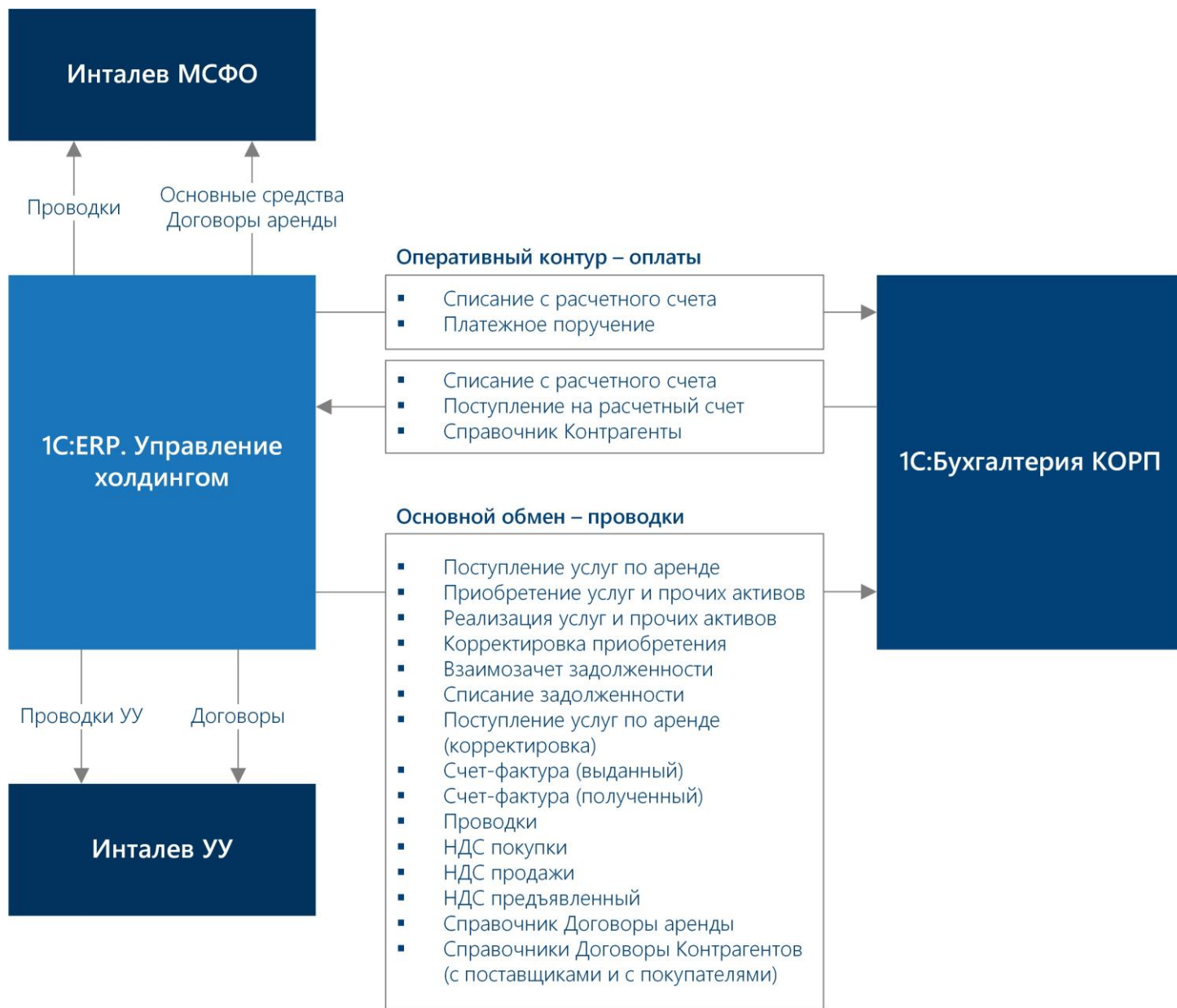
Схема 1. Интеграции между системами
